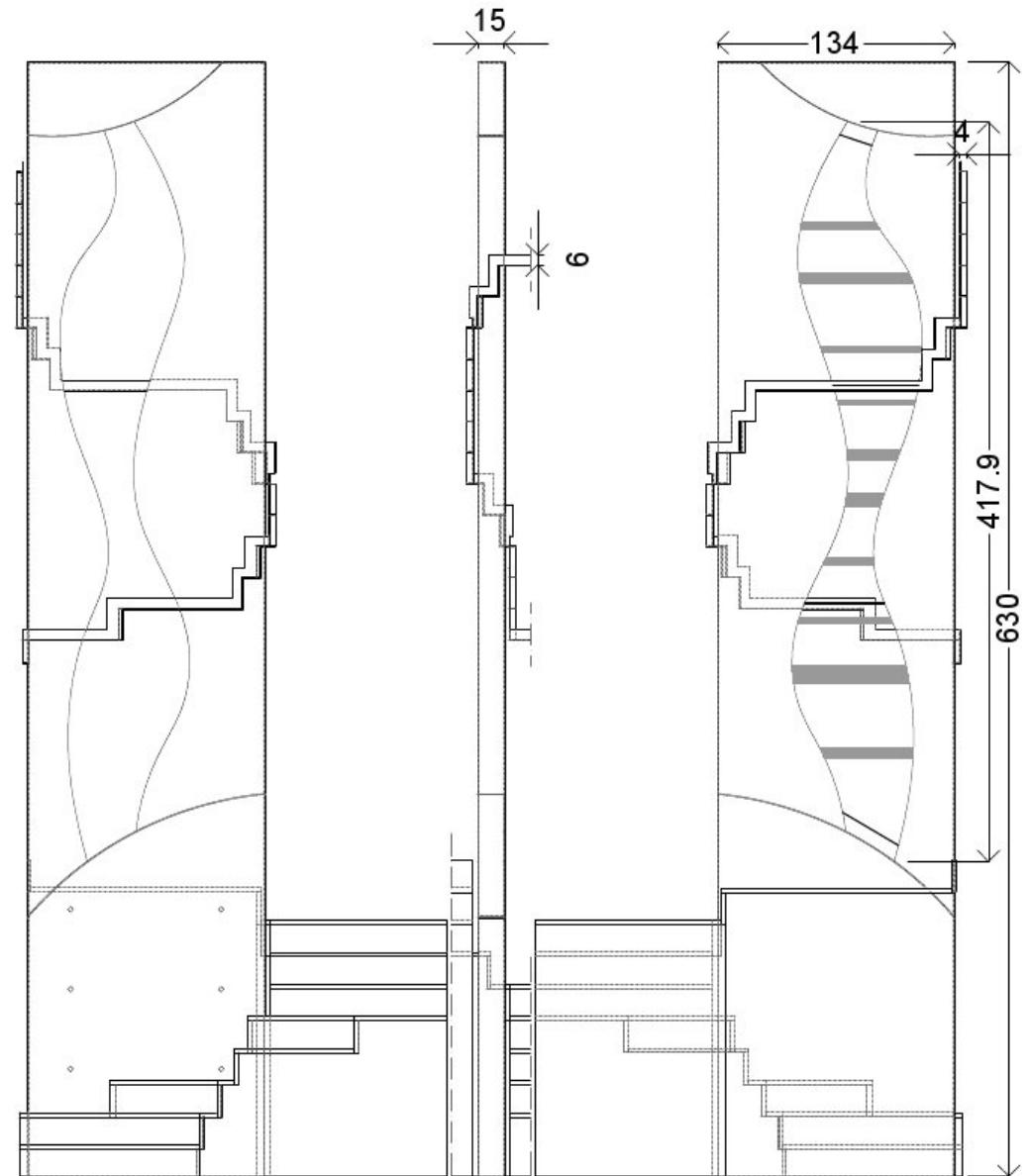
Elemento strutturale corpo scale in acciaio cor-ten
