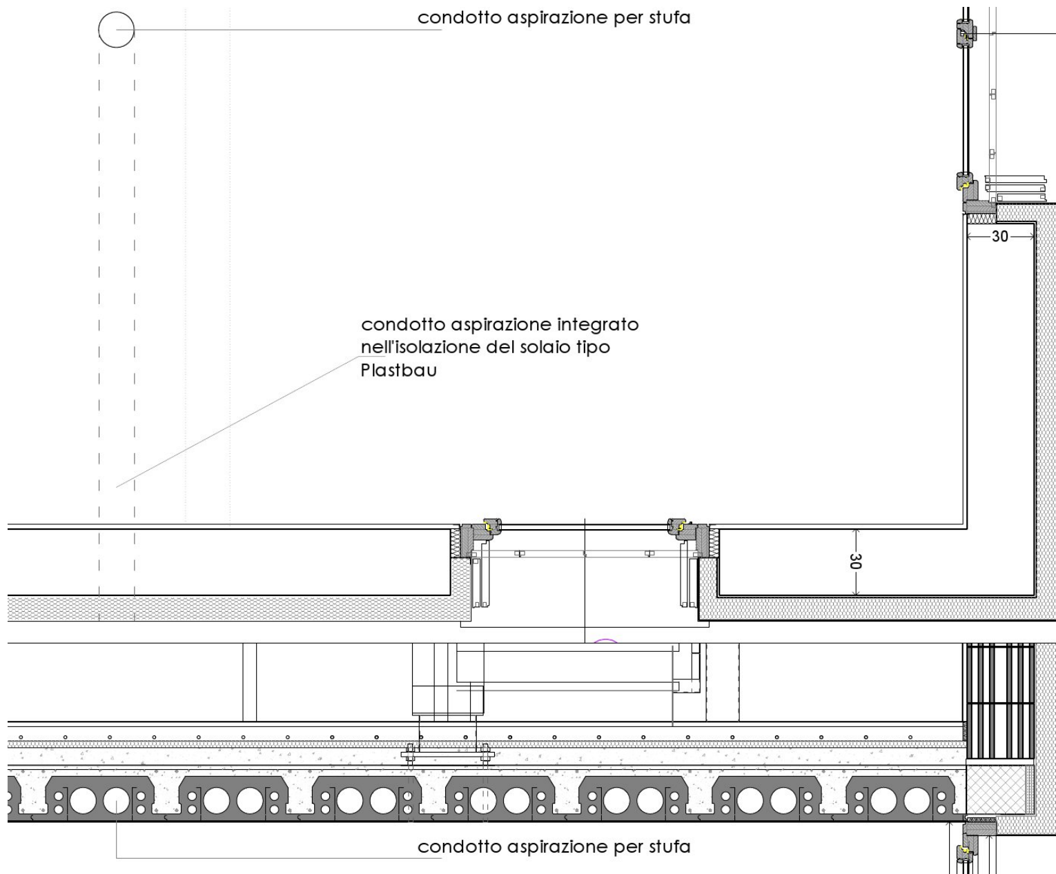
Pianta e sezione solaio tipo plastbau con inserimento condotto aspirazione stufa
