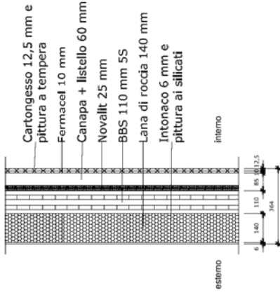
Parete esterna tipo 1
