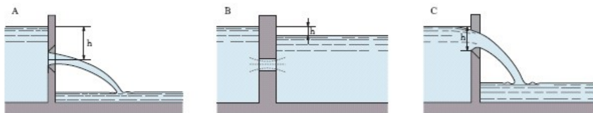
Esempi di foronomia: A – luce a battente libera, B – luce a battente rigurgitata, C – stramazzo libero.
